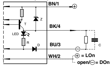
PNP uscita/output
