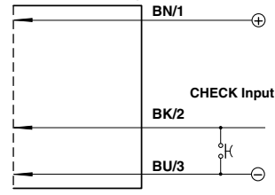
emettitori con check/emitter with check
