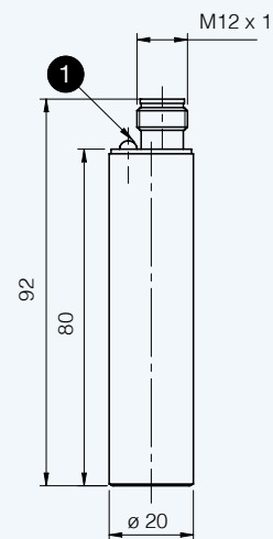
CE*/0*-1E
