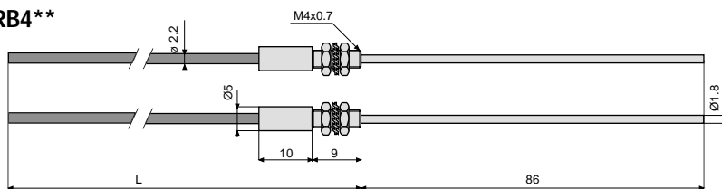
CF/RB6-**
